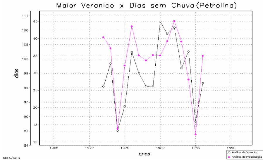
Figura 2 - Ocorrência do número de dias do maior veranico e dos dias sem chuva observados no período de janeiro a abril na Microrregião de Petrolina.
