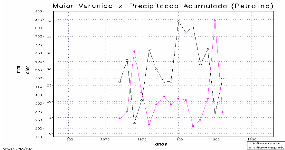
Figura 1 - Ocorrência do número de dias do maior veranico e da precipitação acumulada no período de janeiro a abril na Microrregião de Petrolina.
